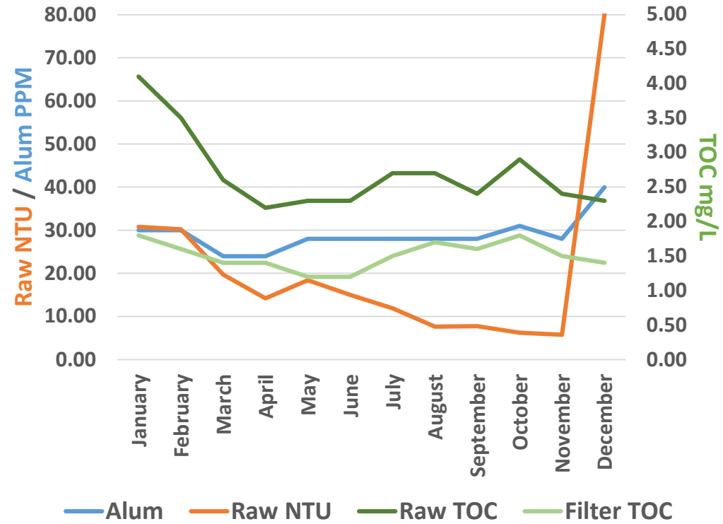
Alum PPM / Raw NTU / TOC Trend 2019
