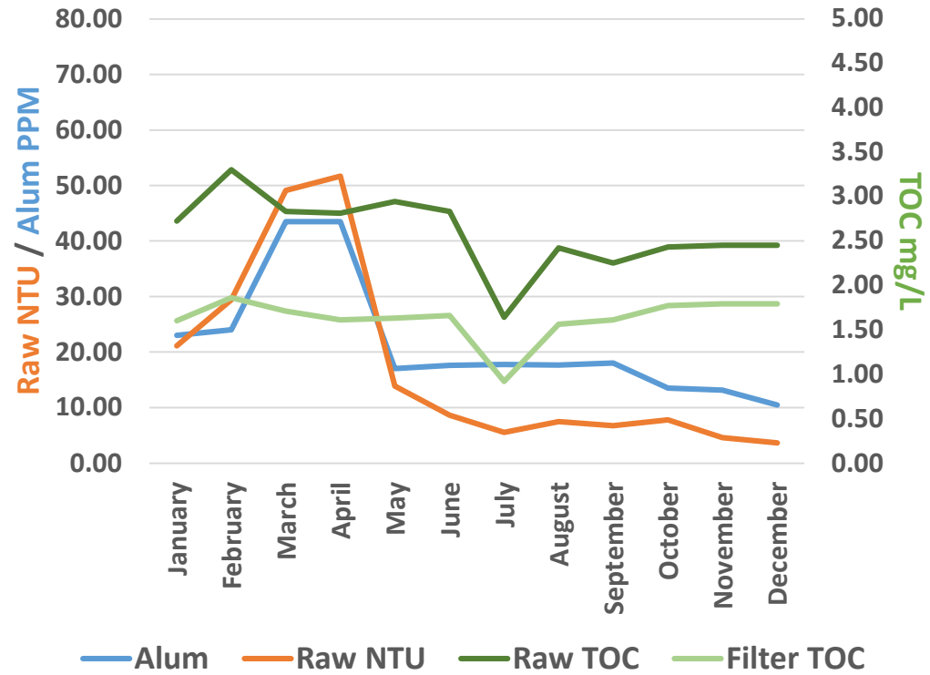
Alum PPM / Raw NTU / TOC Trend 2023
