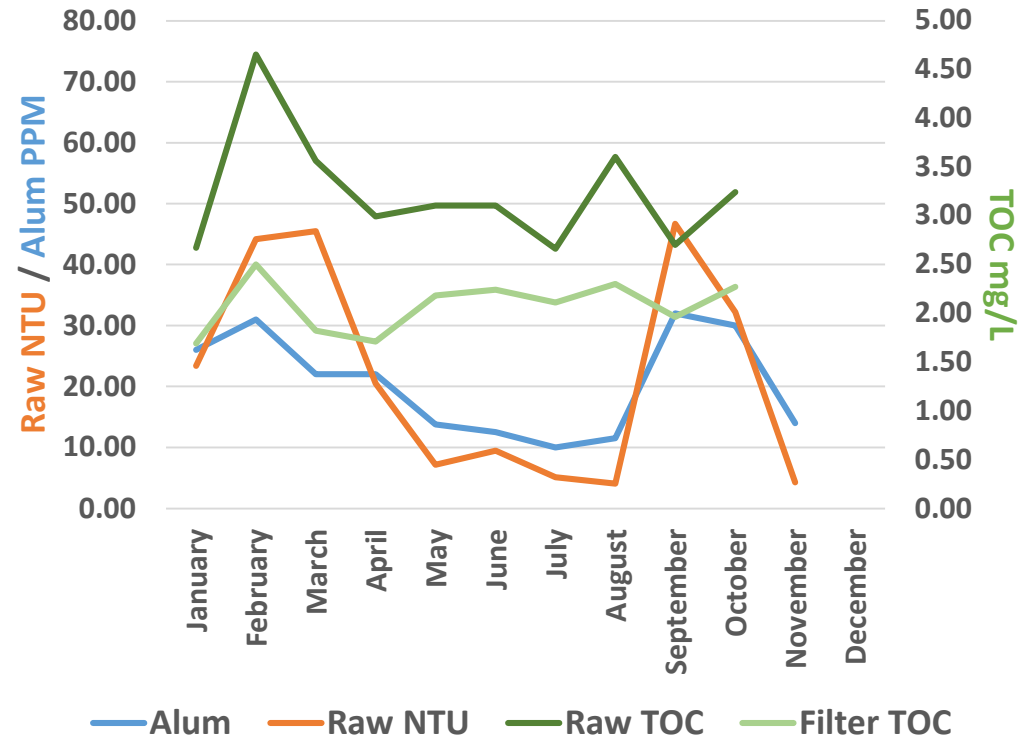
Alum PPM / Raw NTU / TOC Trend 2024
