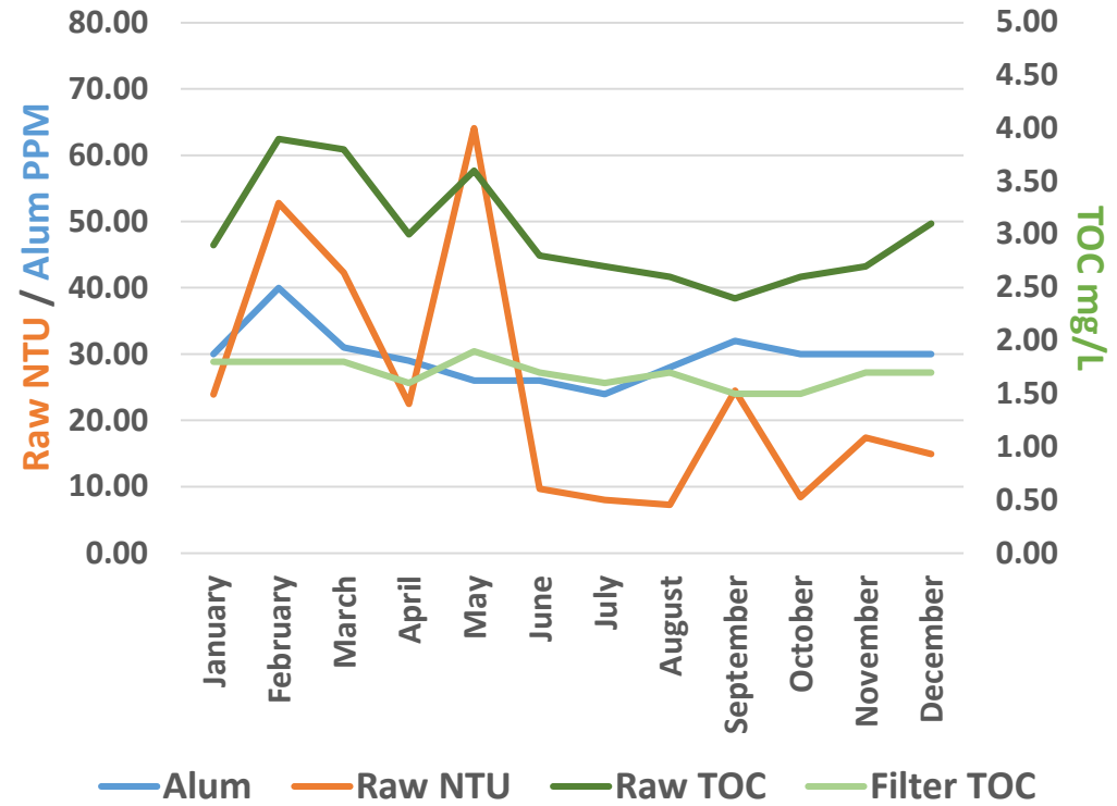
Alum PPM / Raw NTU / TOC Trend 2020
