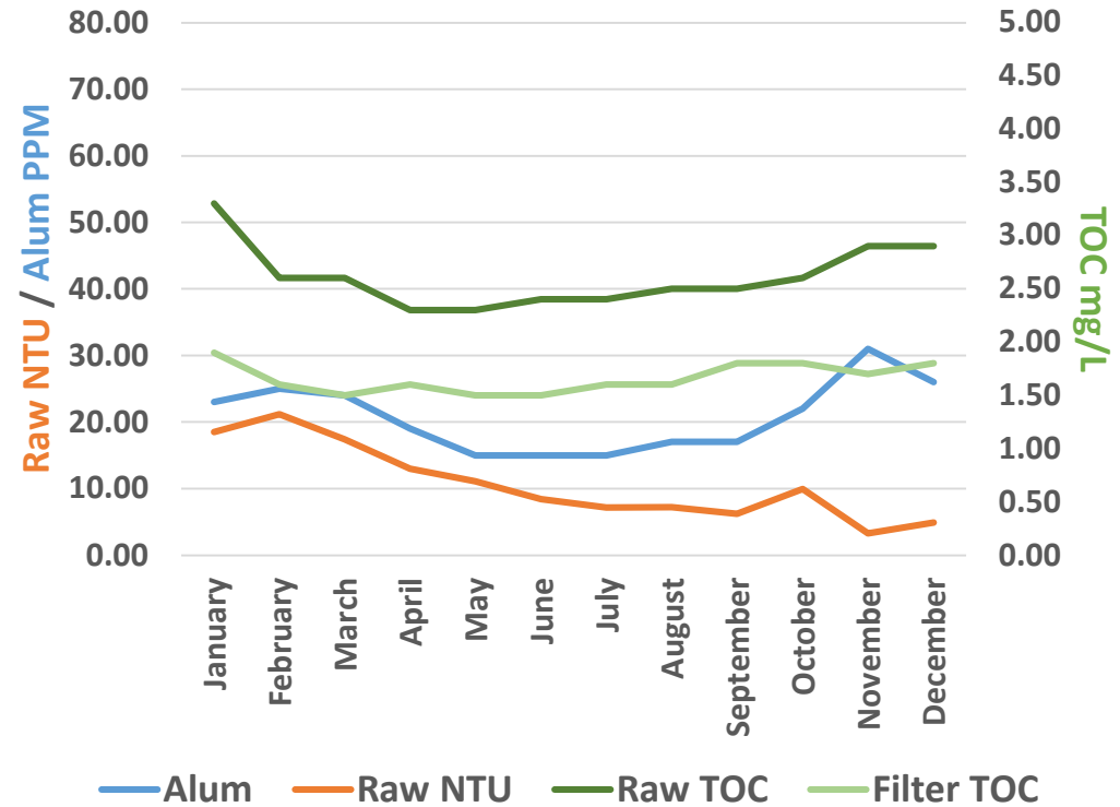
Alum PPM / Raw NTU / TOC Trend 2021
