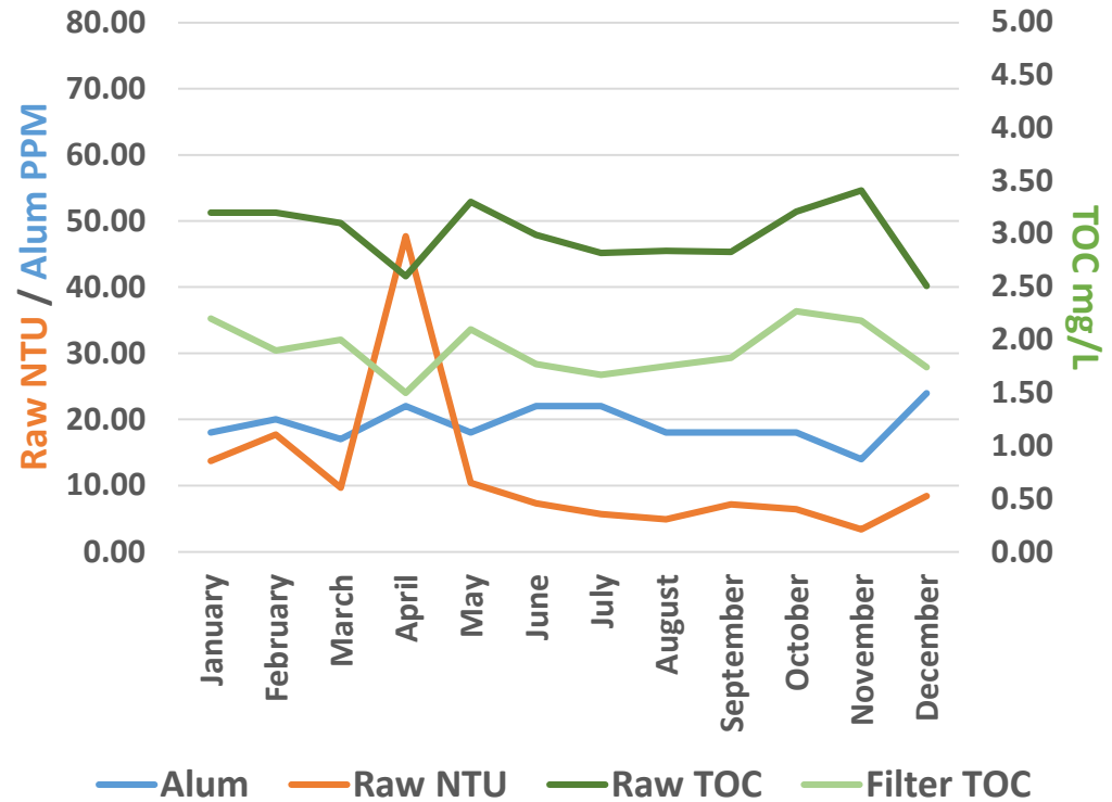
Alum PPM / Raw NTU / TOC Trend 2022
